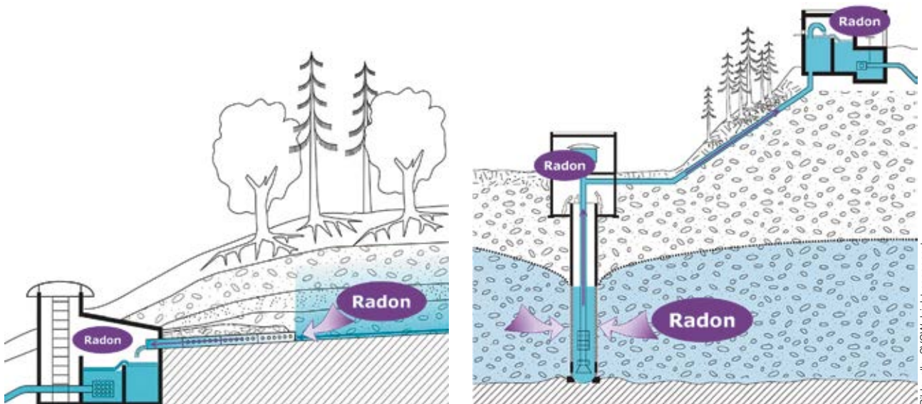
Bild 1 Weg des Radons in die Wasserversorgungsanlage (Quell- und Grundwasser).
