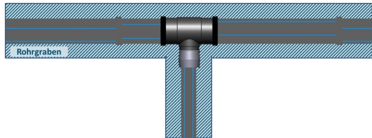
Reduzierter Abzweig mit T-Stück Hauptleitung mit Kurzrohrstück vor dem Abzweig
